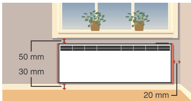
Slika prikazuje propisan minimalni razmak od zidova.
